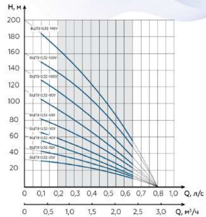
График напорных характеристик
