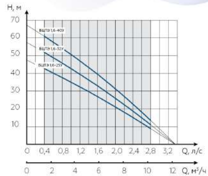
График напорных характеристик
