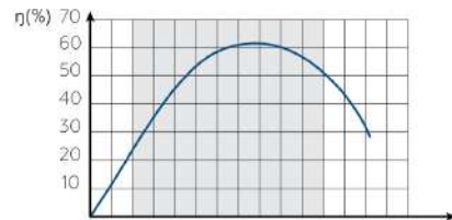
График КПД
