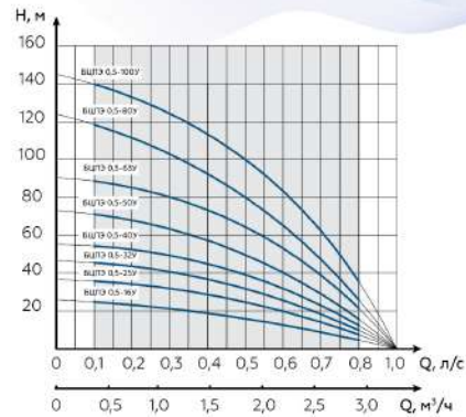
График напорных характеристик
