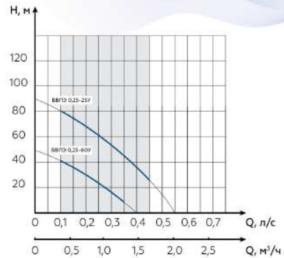
График напорных характеристик
