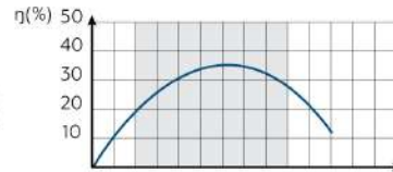
График КПД электродвигателя
